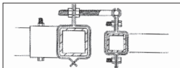
Assemblage de barrière | Gate Assembly Vue du haut | Top View
